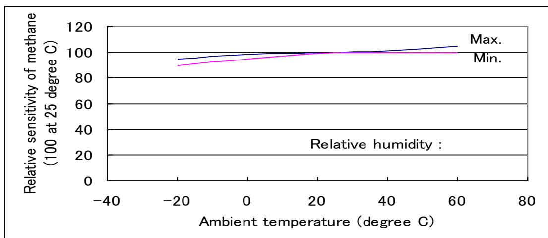
图 4. 温度对甲烷气体的敏感度的影响
