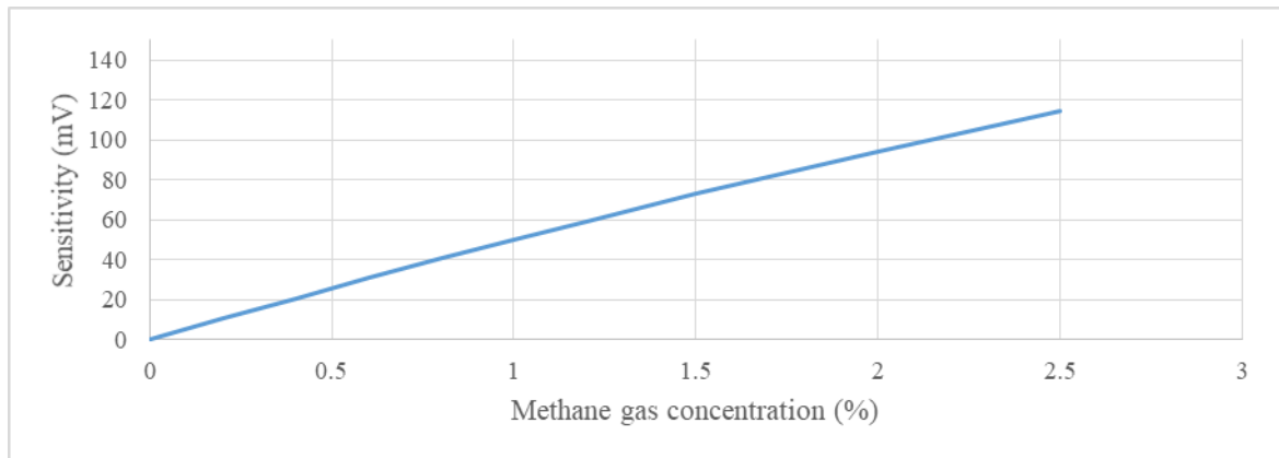
图 2. 到 50%LEL 时甲烷气体的线性度
